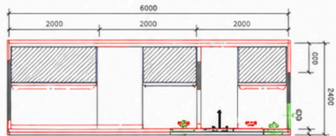
PLANTA BASE
