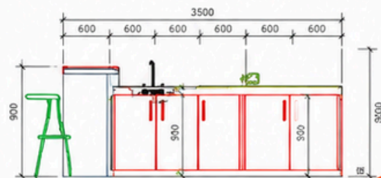
CORTE B-B
